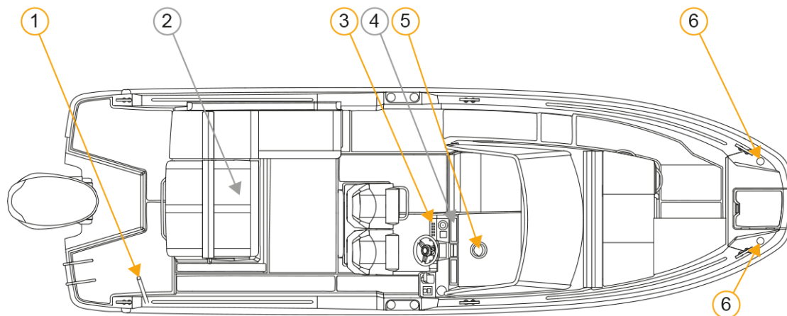
Figure 4.8 Composants du système de navigation
