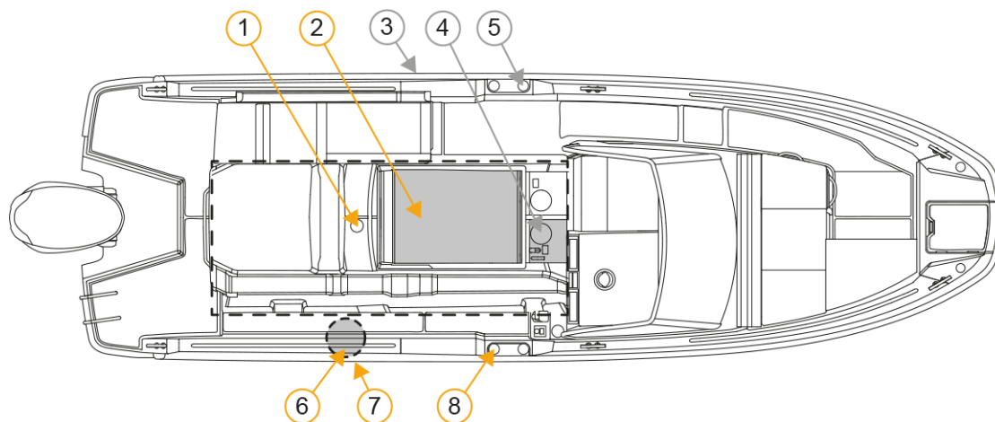
Figure 4.1 Système d'alimentation en carburant
