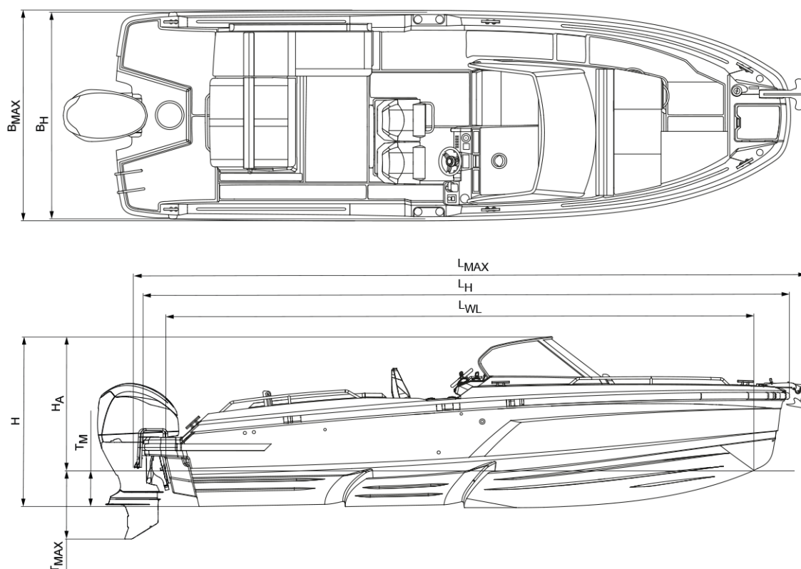
Figure 9.1 Dimensions du modèle Q27 Open
